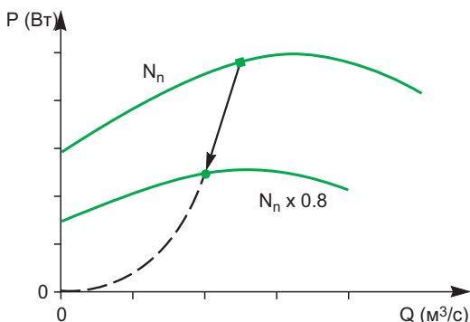
Рис. 17. Характеристика P(Q) центробежного насоса для двух различных скоростей.
