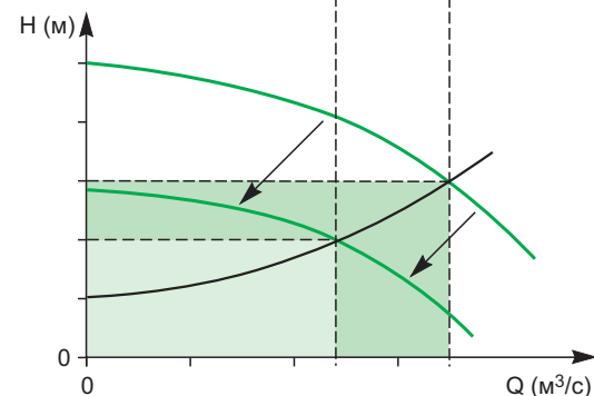
Рис. 18. Регулирование изменения подачи насоса при постоянной и при переменной частоте вращения
