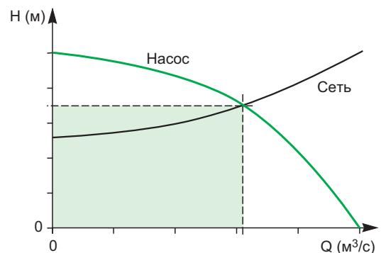
Рис. 8. Рабочая точка насоса в сети.
