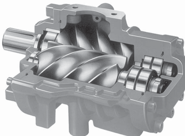
Рис. 44. Пример винтового компрессора
